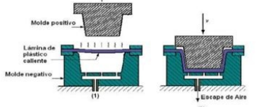
Figura 1.5. Termoformado mecánico(1) 1,1 lámina caliente de plástico se coloca sobre el molde negativo y (2) se cierra el molde para conformar la lámina
